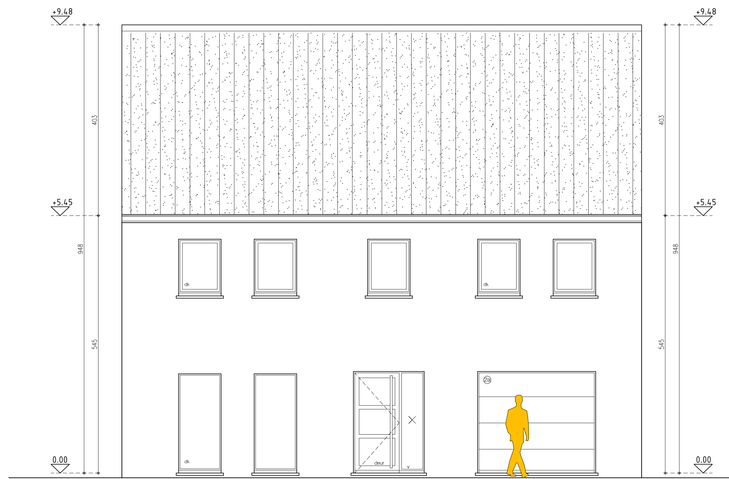
voorgevel
