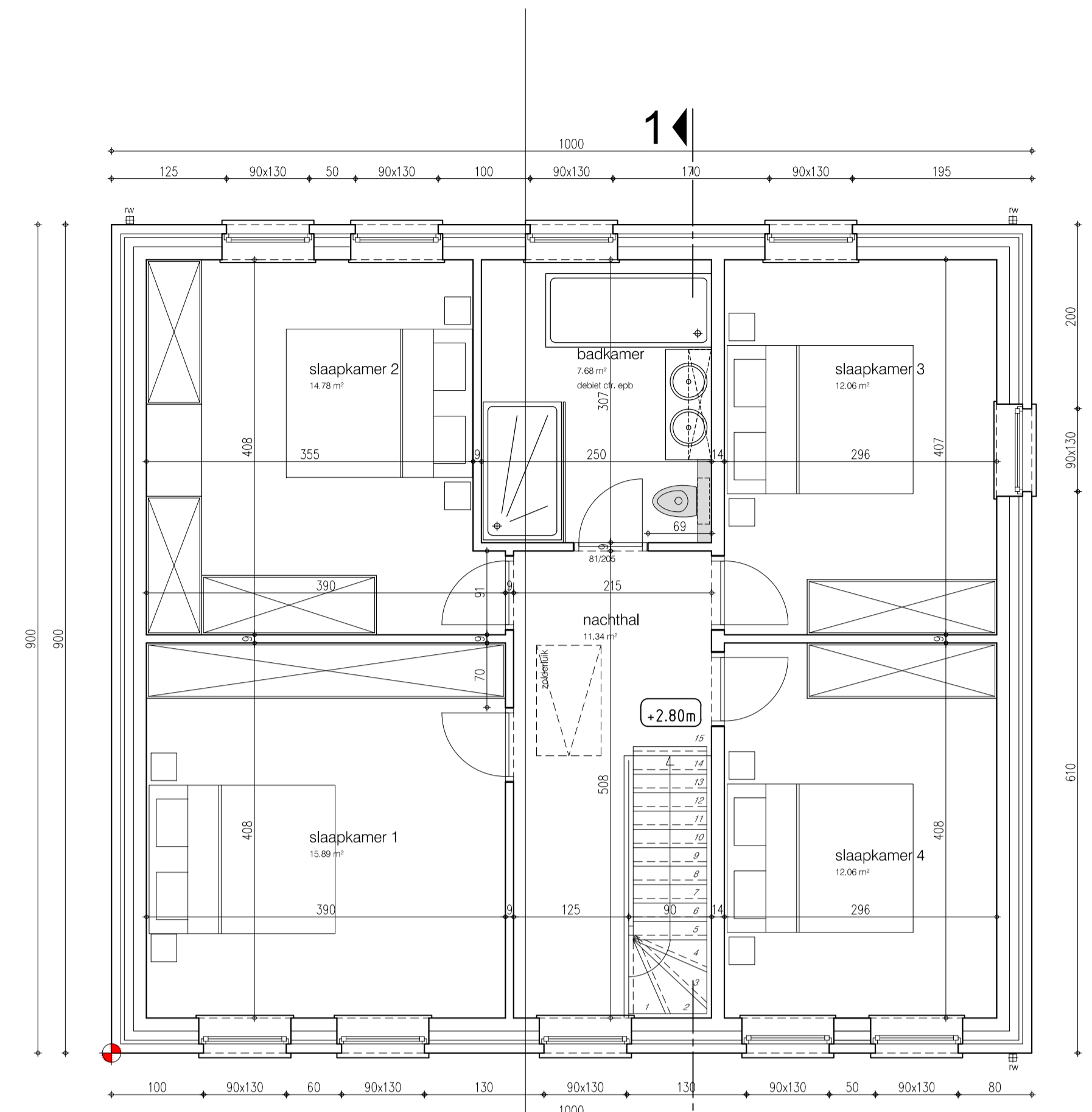
verdiepingsplan
