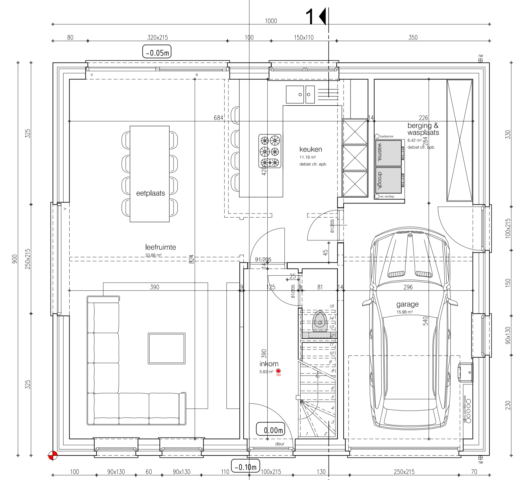
gelijkvloers
